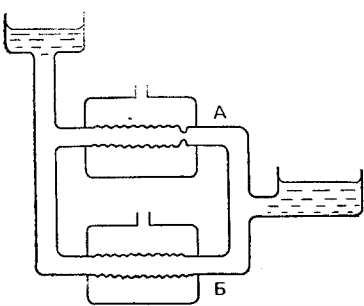
Рис. 4.10. Два сопротивления Старлинга (А и Б), представляющие собой тонкие резиновые трубки, помещенные в камеры. Когда давление в камере больше, чем в конечном отрезке трубки (А), расход жидкости не зависит от давления оттока. В противоположном случае (Б) расход жидкости определяется разностью давлений притока и оттока
